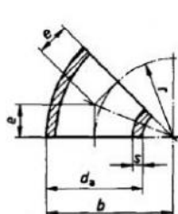
45° elbow
