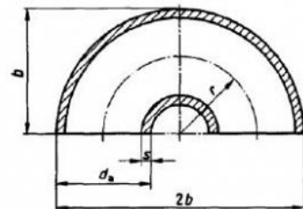
180° bend
